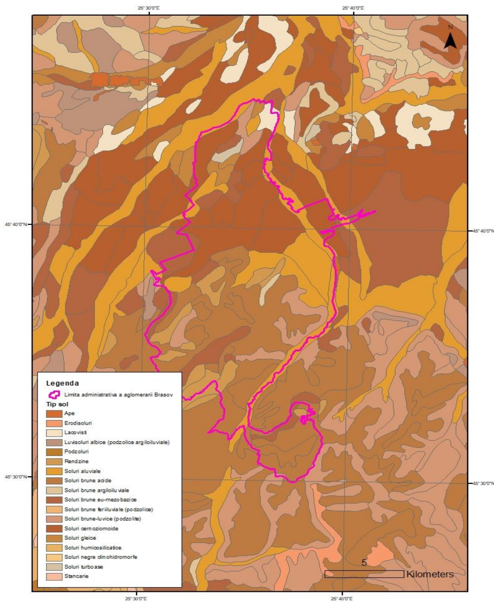
Figura 5 - Tipurile de sol identificate la nivelul municipiului Brașov (MULTIDIMENSION, 2022)
